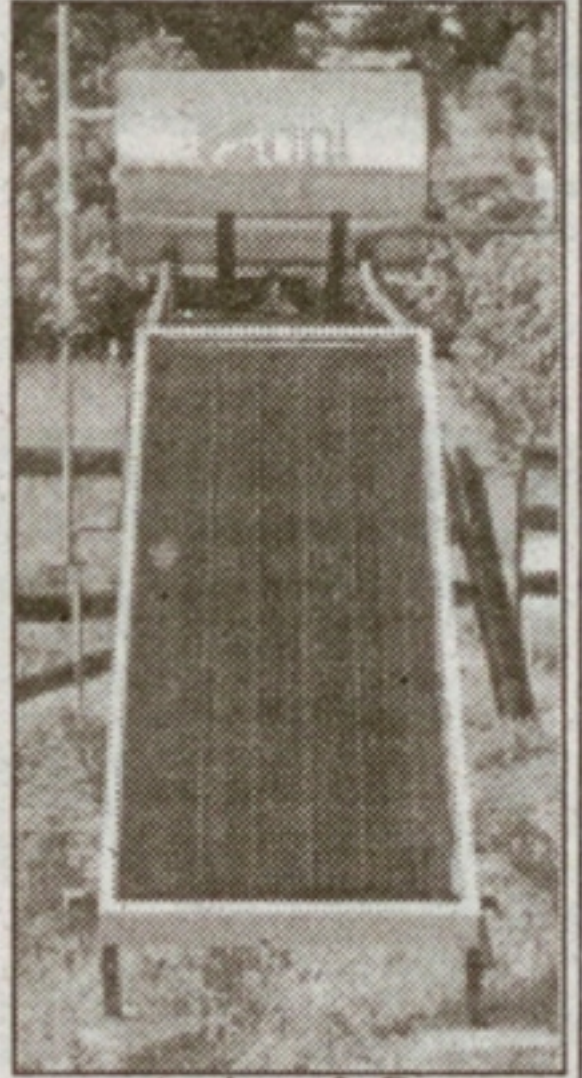
अग्नी सोलर सिस्टिम्स कंपनीचा 'मिनी सोलर हीटर'
